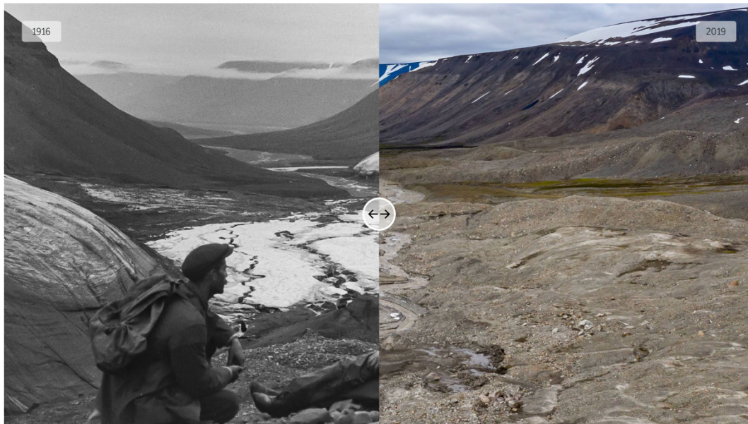
Rolterdalen nå Svalbard fotografert i 1916 og i 2019
