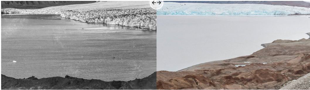
Tempelfjorden på Svalbard fotografert i 1908 og i 2019 NORSK POLARINSTITUTT/ERIK SCHYTT HOLMLUND
