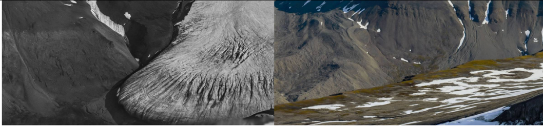
Rieperbreen på Svalbard fotografert i 1914 og i 2019 NORSK POLARINSTITUTT/ERIK SCHYTT HOLMLUND
