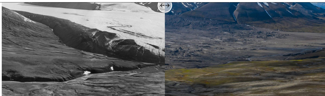
Drønbreen på Svalbard fotografert i 1925 og i 2019 NORSK POLARINSTITUTT/ERIK SCHYTT HOLMLUND
