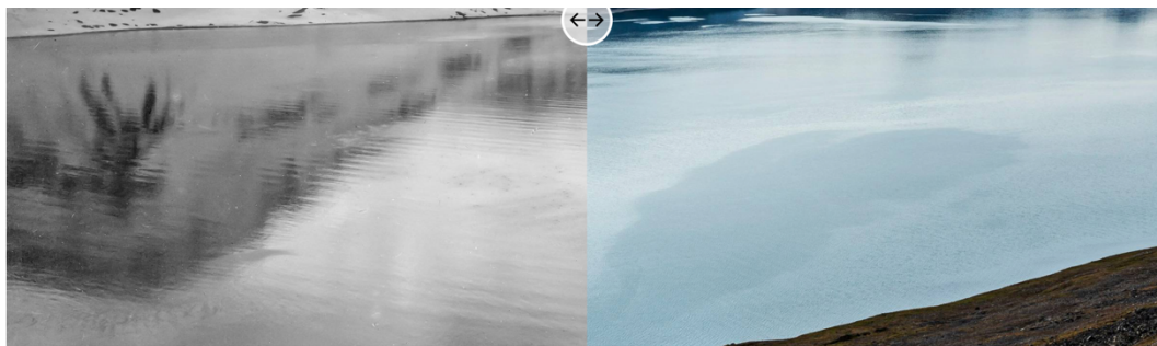
Trygghamna fotografert i 1908 og i sommer NORSK POLARINSTITUTT/ERIK SCHYTT HOLMLUND
