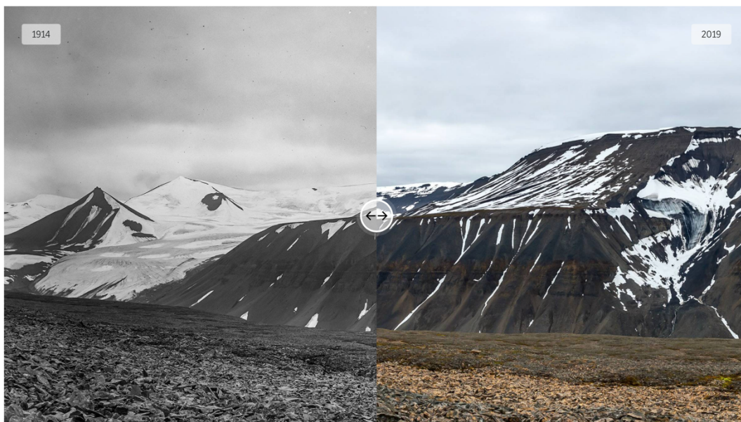
Breinosa på Svalbard fotografert i 1914 og i 2019 NORSK POLARINSTITUTT/ERIK SCHYTT HOLMLUND
