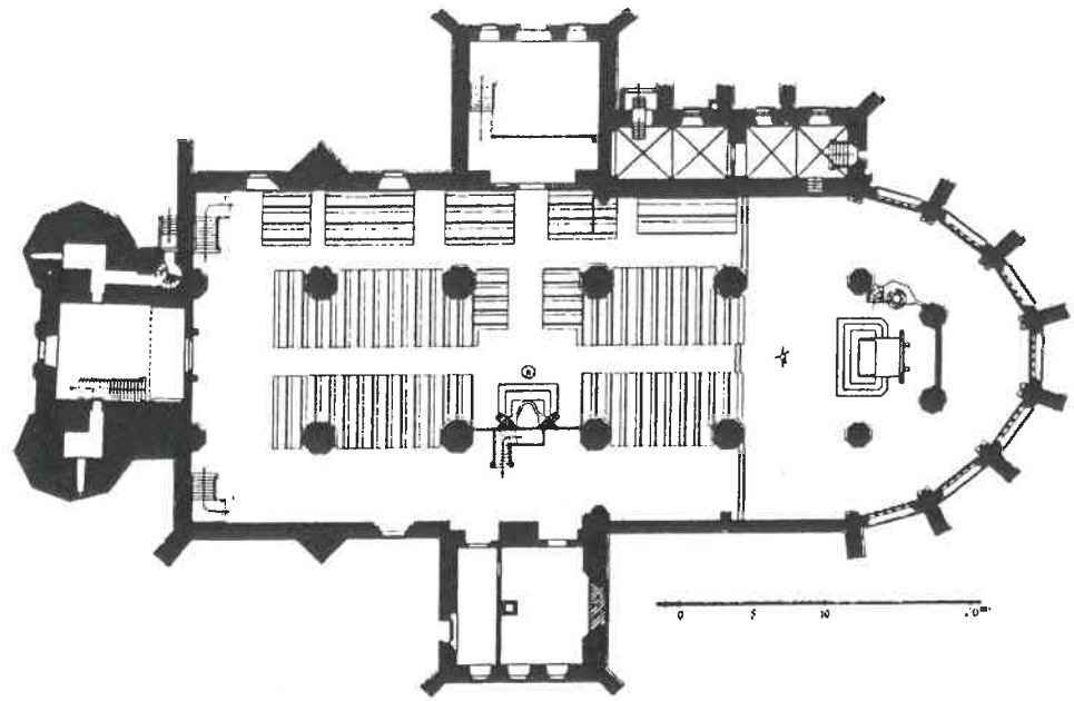
Abb. 105 - 106 FÜRSTENWALDE/SPREE, QUERAUSRICHTUNG DER MITTELALTERLICHEN DOMKIRCHE
