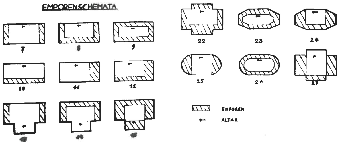
Abb.2 Einteilung der Querkirchen nach Ilse Dött, 1955
