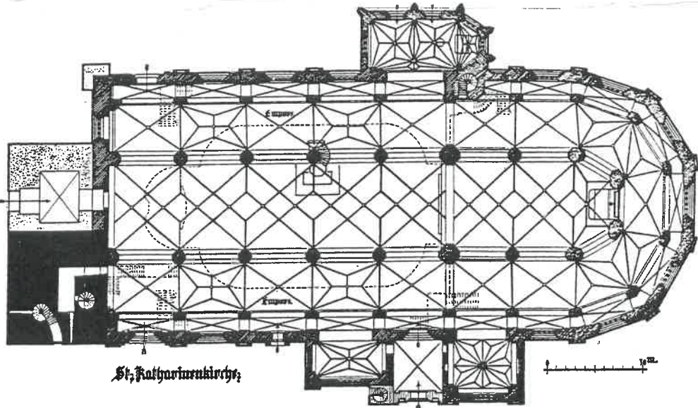
Abb. 89 - 90 BRANDENBURG/HAVEL, QUERAUSRICHTUNG DER MITTELALIERLICHEN ST.KATHARINENKIRCHE
