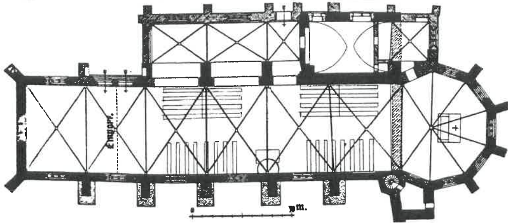
Abb. 93 - 94 BRANDENBURG/HAVEL, QUERAUSRICHTUNG DER MITTELALIERLICHEN ST. JOHANNESKIRCHE
