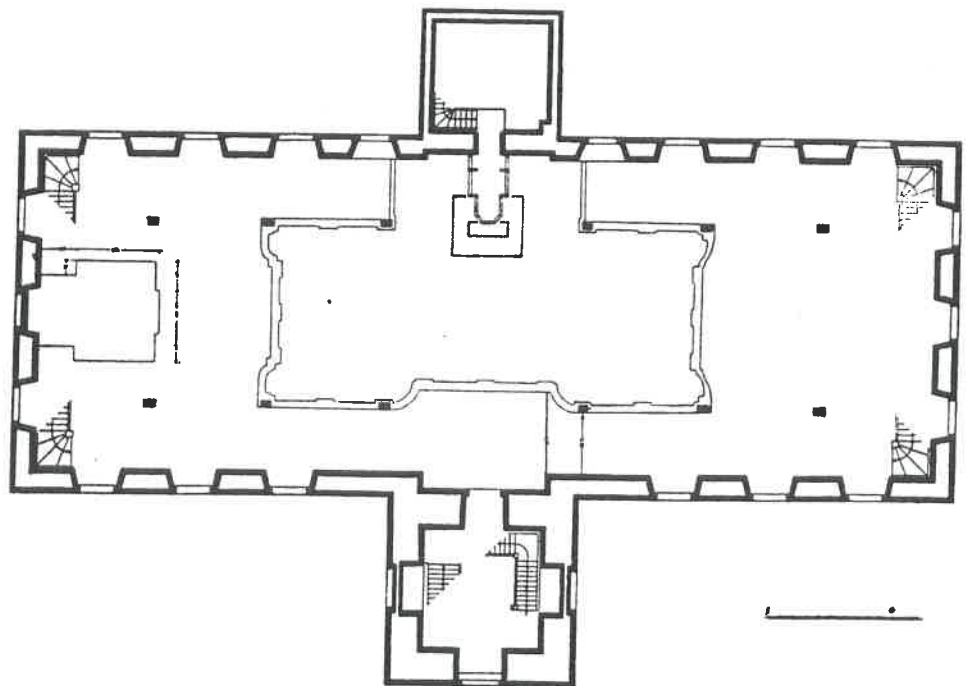
Abb. 68 und 69 ZOSSEN, Querkirche von 1734/35
