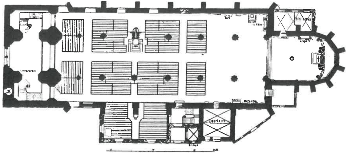
Abb. 102 - 104 BERLIN ST.MARIENKIRCHE, Grundriss und Innenansicht des querorientierten Kirchenraumes vor dem Umbau von 1954. Aussenansicht mit Südkapelle.
