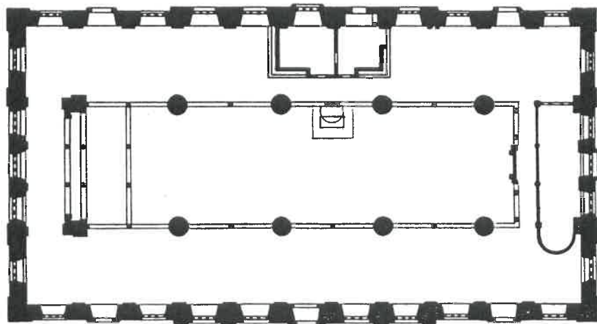
Abb. 41 Ursprünglicher Quergrundriss
