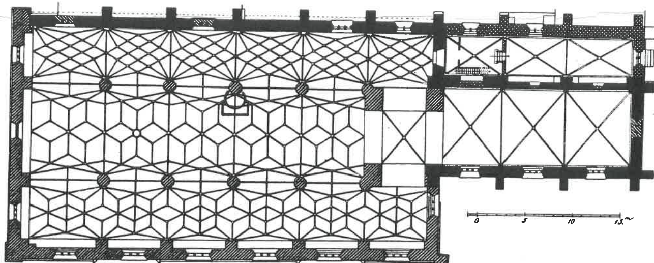
Abb. 97 - 98 FRANKFURT AN DER ODER, QUERAUSRICHTUNG DER MITTELALTER- LICHEN FRANZISKANERKLOSTERKIRCHE
