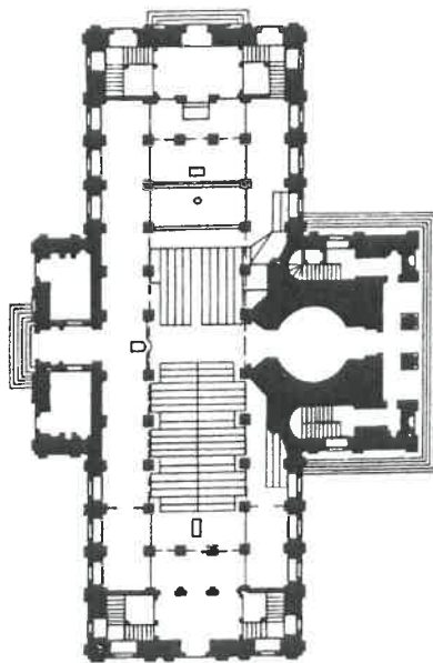
Abb. 46 Grundriss des längsgerichteten Kirchenraumes vor 1817
