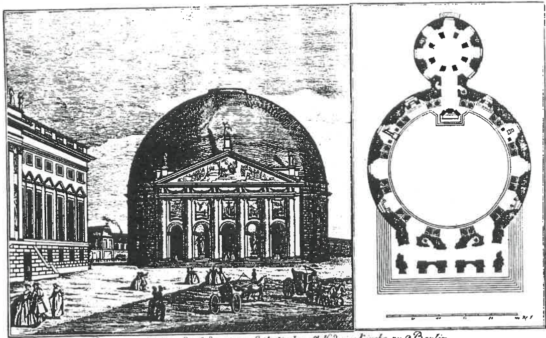
Prospect und Grundriß der neuen katholischen Hedwigs Kirche zu Berlin.
