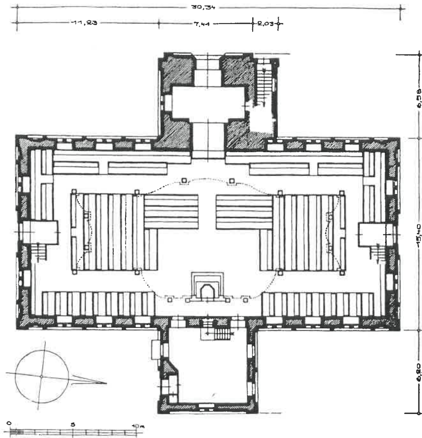
Landsberg. Konkordienkirche. Grundriß
