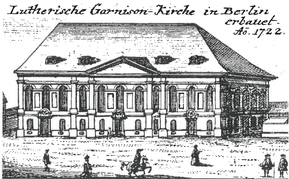
Abb. 40 Ansicht um 1850
