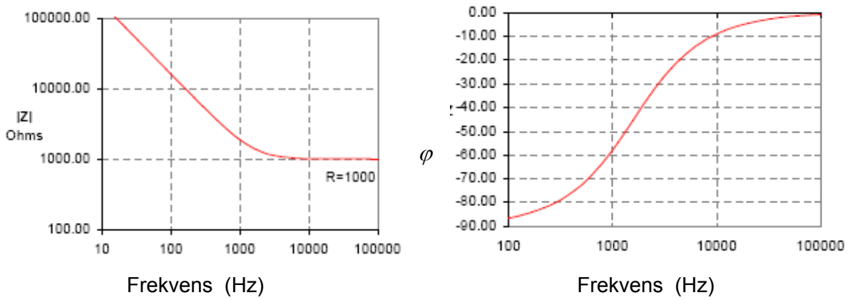
Figur 2.5: Bode plott av impedans
